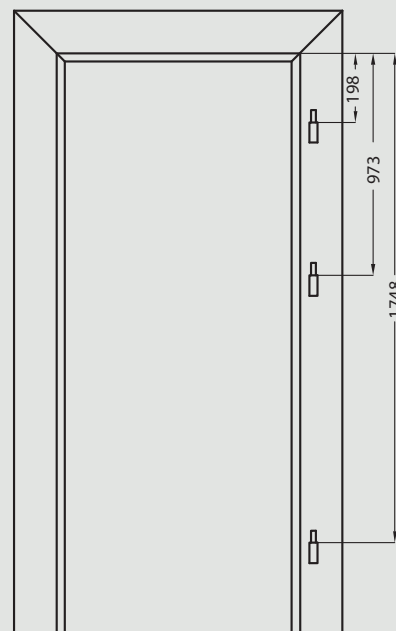
Vodorovný prierez
