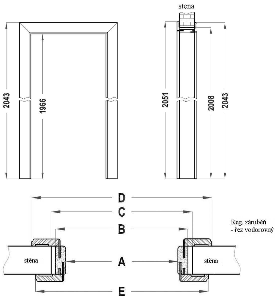
Obrázek 3. Pohled na regulovanou zárubeň a její průřez
