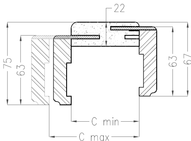
Obrázek 1. Přizpůsobení regulovatelné zárubně do tloušťky stěny
