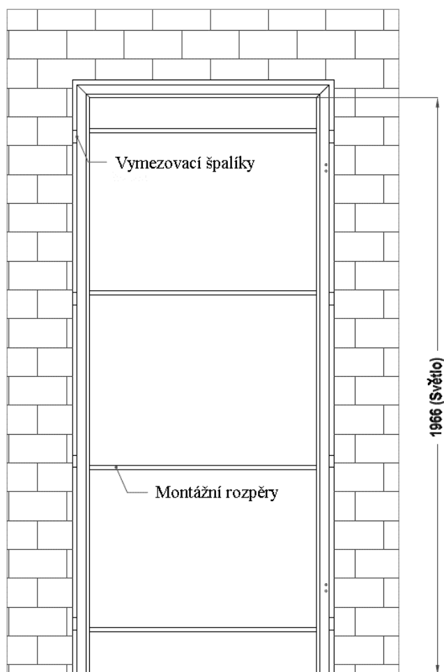
Obrázek 2. Montáž regulovatelné zárubně do stěny
